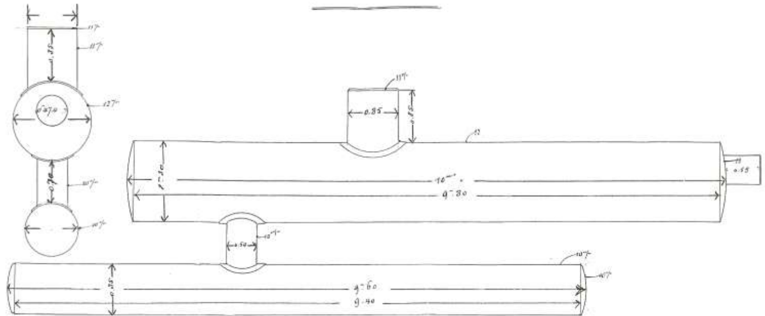
Figuur 3: plan van stoomketel die voor de verwarming instond.
