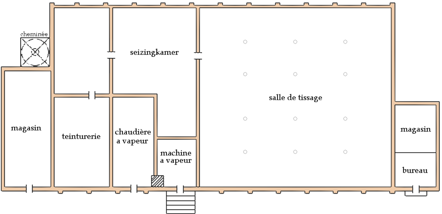
Figuur 5: plattegrond van de nieuwe fabriek van d'Heygere,
