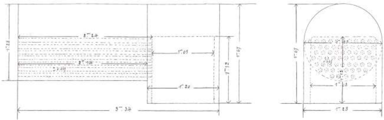
Figuur 2: Technisch plan van de stoommachine die werkvloer moest verwarmen.
